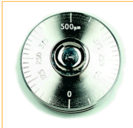
Elcometer 3230 Nassfilmrad
