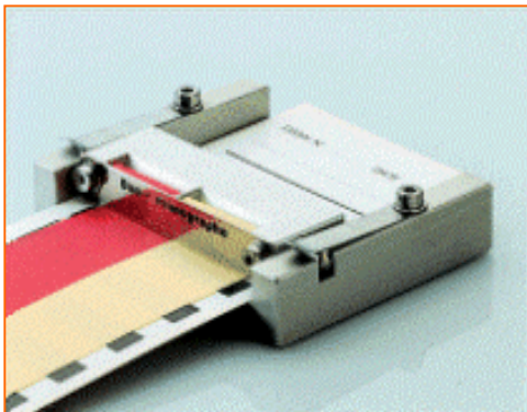
Aplicadores Doctor Blade de varias películas Elcometer 3800 v 3805
